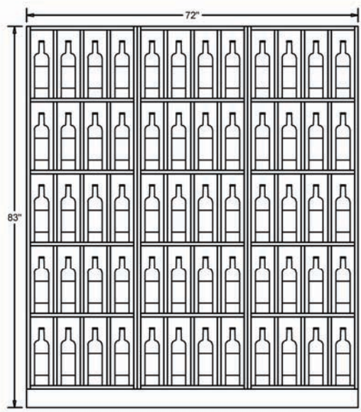
ELEVATION -L-
