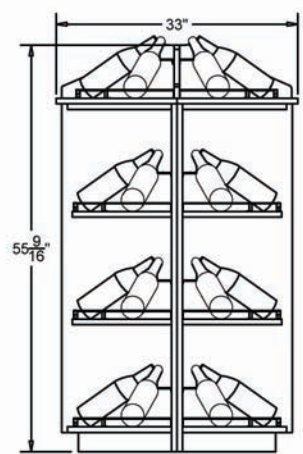
ELEVATION -C-
