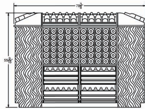
ELEVATION -J-
