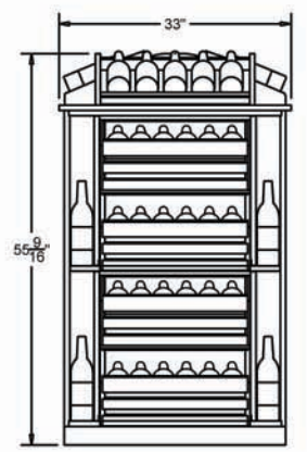
ELEVATION -K-
