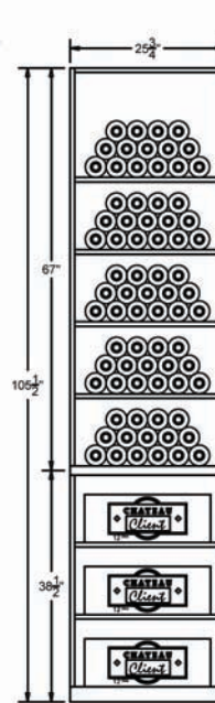
ELEVATION -C-
